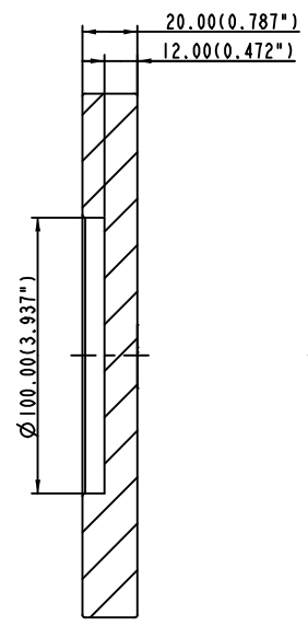
Section A-A
